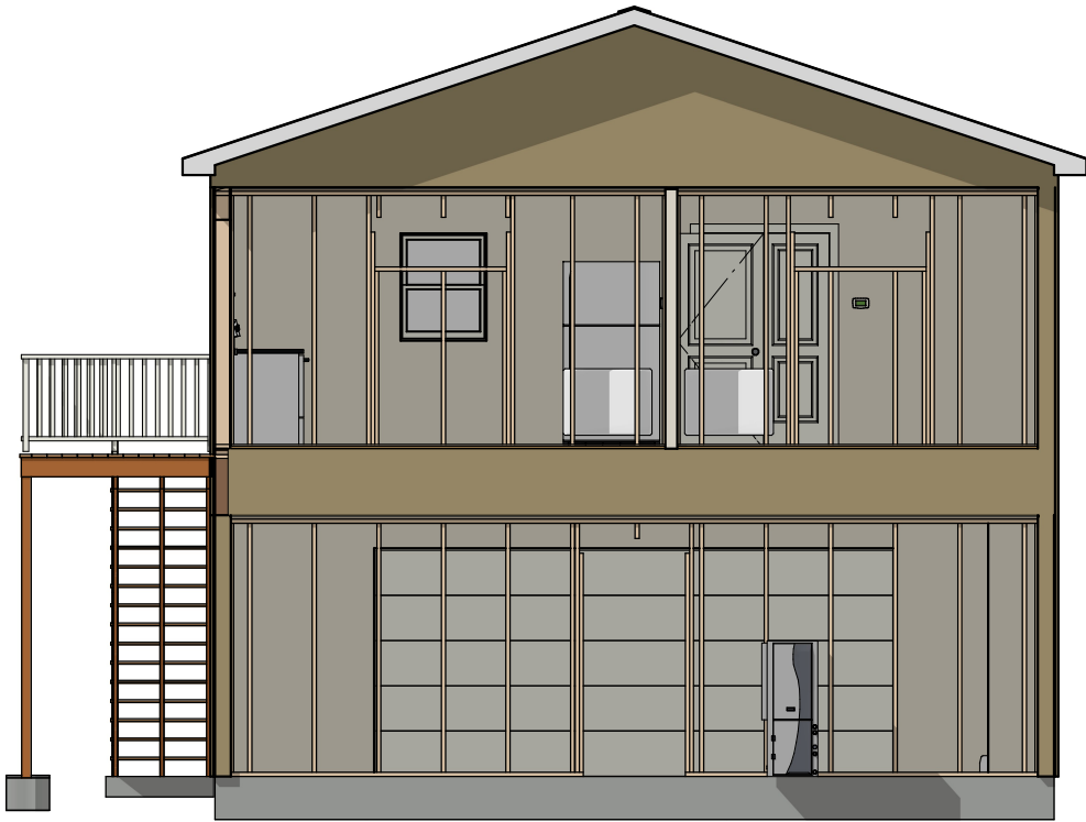
Elevation 4
